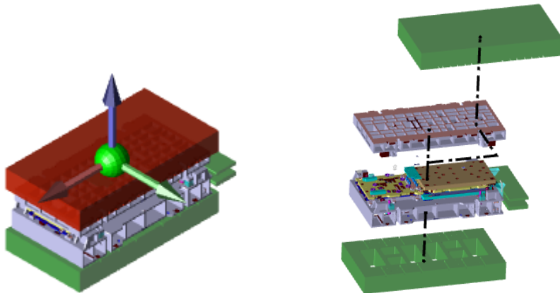
< 파트 분해 >
